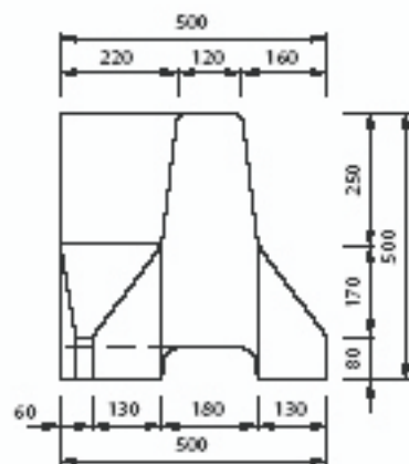
POHLED ČELNÍ
