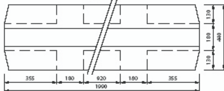
PŮDORYS
